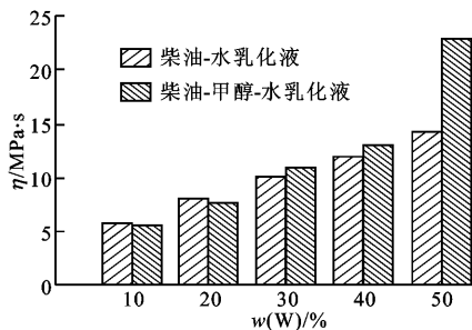
图5 w(E)=8\% 时2种乳化液的黏度与含水率的关系
