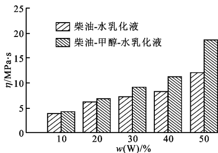
图3 w(E)=4\% 时2种乳化液的黏度与含水率的关系
