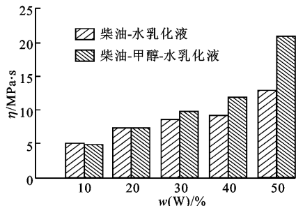
图4 w(E)=4.8\% 时2种乳化液的黏度与含水率的关系
