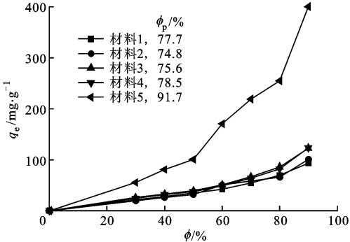
图 5 材料饱和吸附量随相对湿度的变化规律
