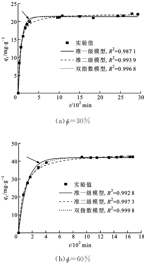
图 3 不同动态吸附模型的吸附动力学曲线对比
