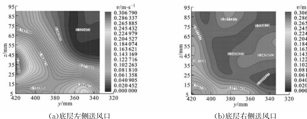
图10 冷藏室第四层间室送风口中心平面内速度等值线分布图
