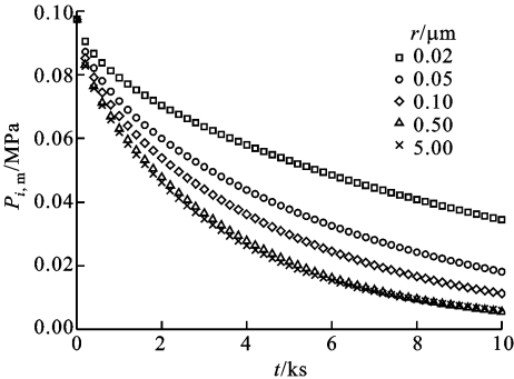
(a)CH 4 的扩散过程
