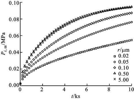
(b)Ar 的扩散过程
