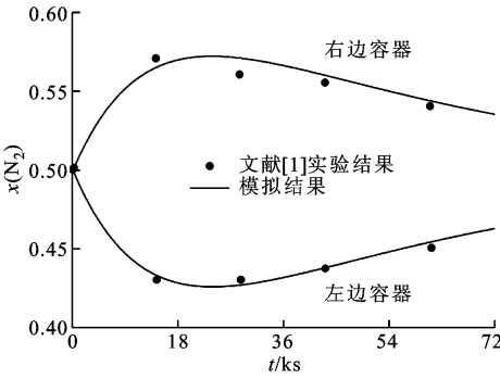
(b) \text{N}_2 的摩尔分数随时间的变化
