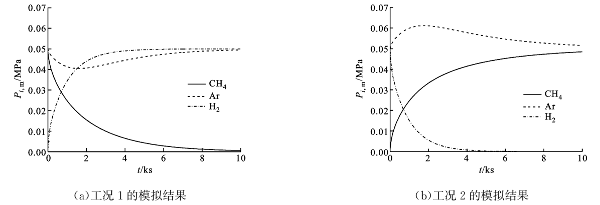
图 5 三元混合气体在多孔介质内扩散过程的模拟结果
