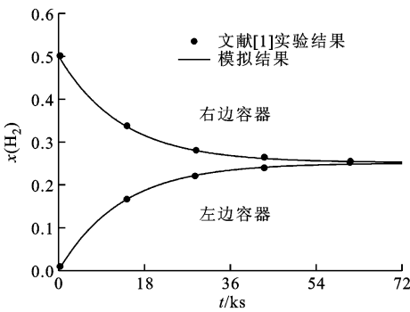
(a) \text{H}_2 的摩尔分数随时间的变化
