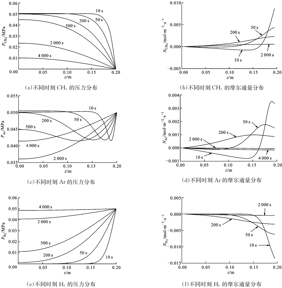
图 6 工况 1 各组分在不同时刻的压力和摩尔通量分布
