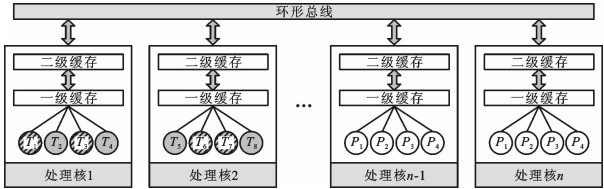
(a)OpenMP 内置的 Compact 映射模式
