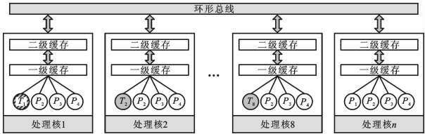
(b)OpenMP 内置的 Scatter 映射模式
