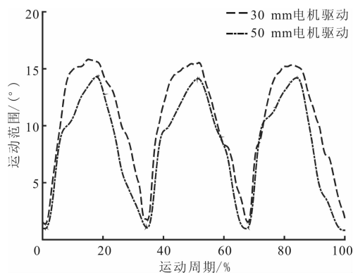
图7 指尖力测量结果
