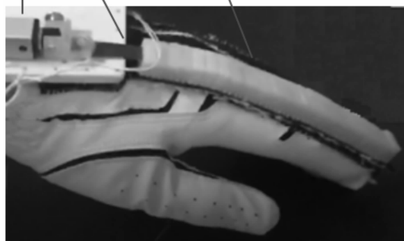
图1 多段连续结构外骨骼手功能康复机器人
