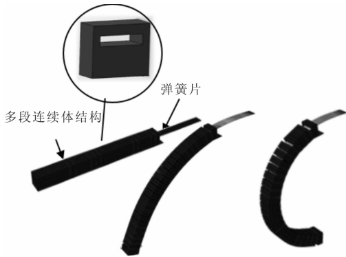
图 2 多段连续体弯曲示意图
