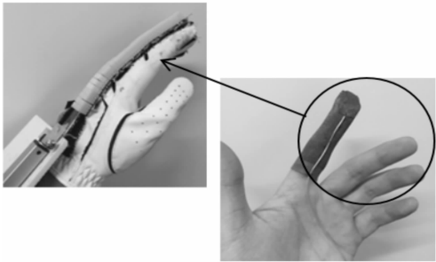
图 6 测量指尖力的实验装置
