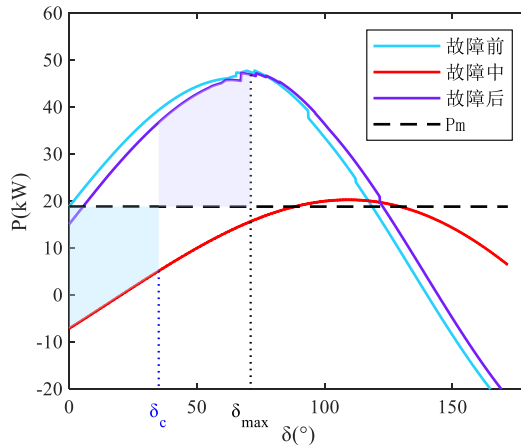
图 17 含直流的EAC曲线
