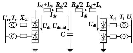
图1 一次系统机电暂态模型图
