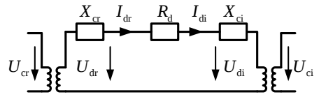
图3 直流模型一次侧稳态模型
