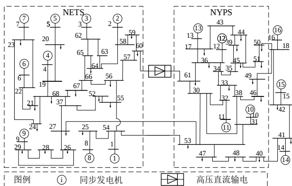
图7 16机-68节点系统
