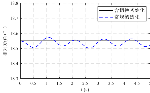
图 11 初始化后等效功角曲线
