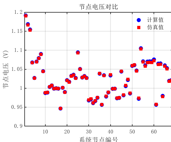
图13 切除故障后节点电压仿真值与计算值对比图
