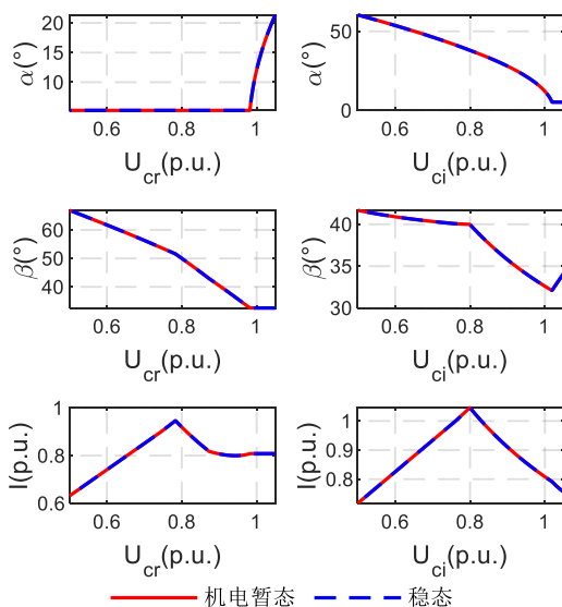
图5 DM各电气量对比图
