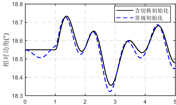
图 12 切除故障后等效功角曲线
