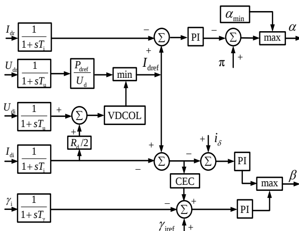
图2 DM模型示意图
