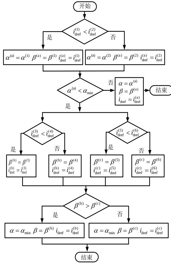
图4 DM模型控制模式逻辑判断图
