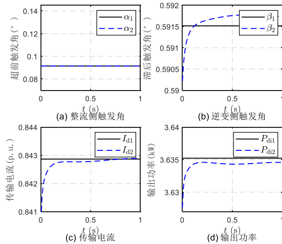
图10 \lambda = 3.4 各电气量对比示意图
