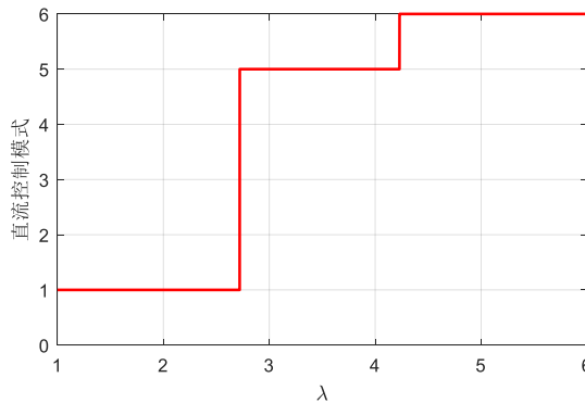
图8 直流模式随负荷切换结果图
