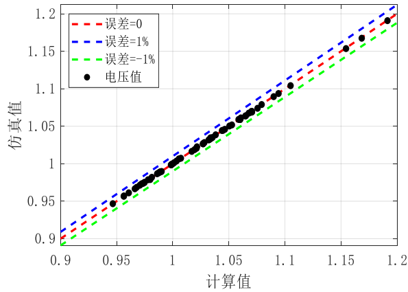
图 16 切除故障后节点电压误差分析
