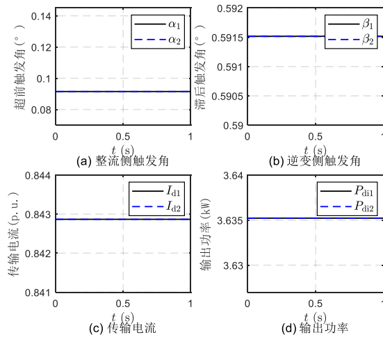
图9 \lambda = 1 各电气量对比示意图
