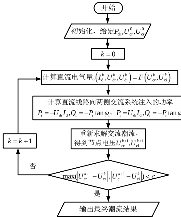
图 6 含直流系统的初始化求解方法
