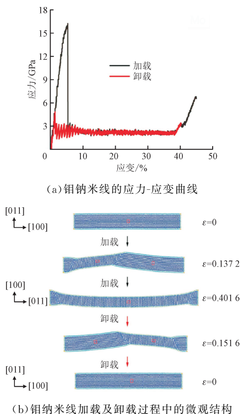
图4 钼纳米线的超弹性行为及其微观结构演化 [11]
