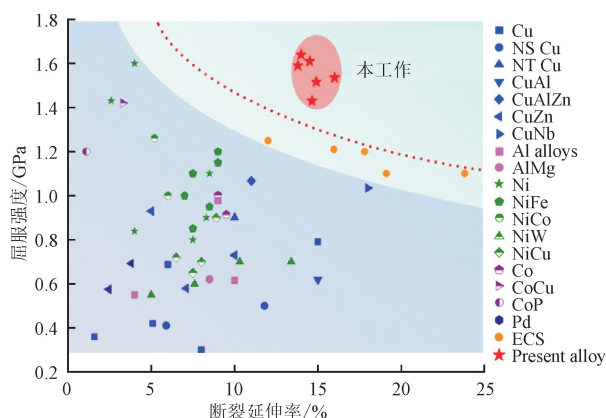
(b)成分起伏纳米晶合金与报道过的纳米晶单相合金对比 图 10 成分起伏纳米晶合金超高强塑性 [35]
