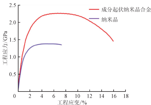
(a) 成分起伏纳米晶合金与传统纳米晶 Ni 的力学性能对比
