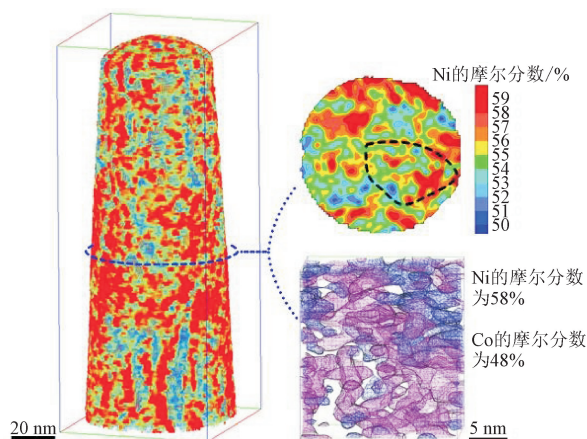
图8 合金内部成分起伏波动程度的三维原子探针结果 [35]
