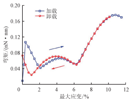
(a) 钛酸钡薄膜的最大应变-弯矩曲线
