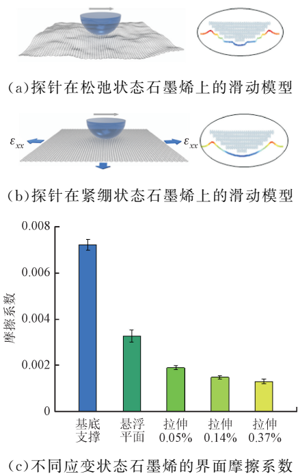
图2 应变调控实现超润滑 [7]
