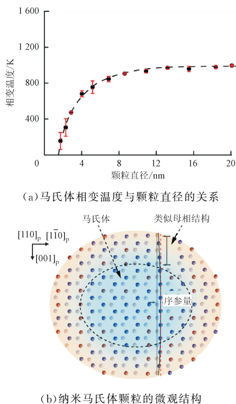
图5 B2 至 B19 马氏体相变的尺度效应及相变序参量在表面附近的连续转变 [15]
