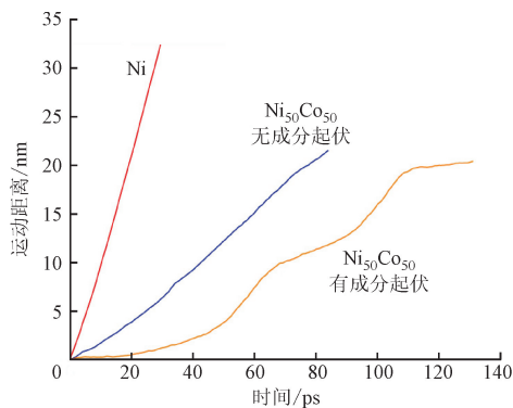
图 9 成分起伏波动程度对位错运动行为的影响 [35]
