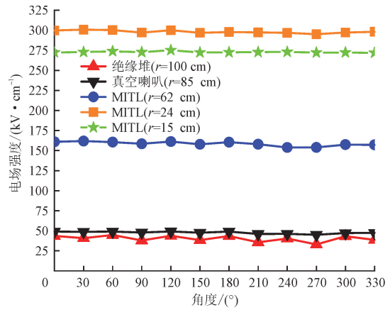
(a) 不同位置的电场
