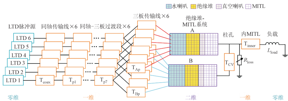
(a) 多路并联 LTD 装置二维传输线电路模型
