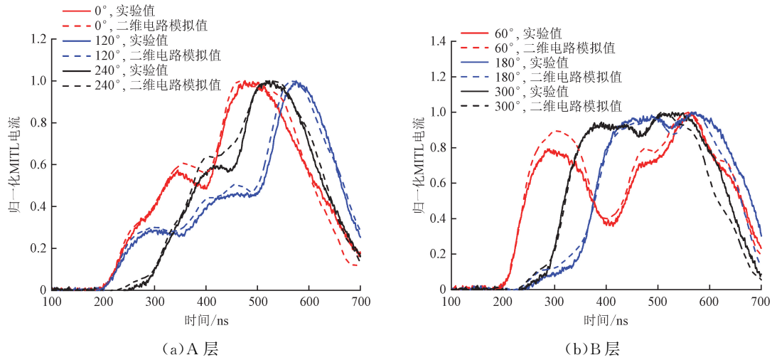
图10 不同角向位置的归一化 MITL 电流波形
