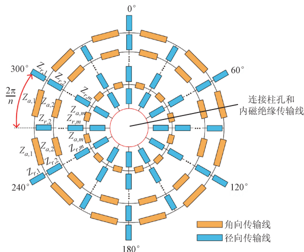
(b) A 层绝缘堆-MITL 二维电路模型
