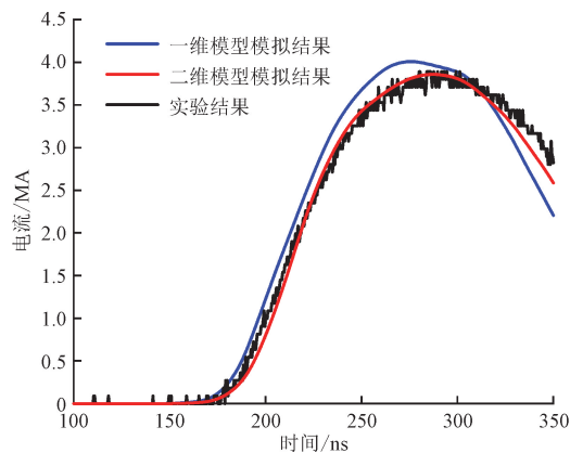
图 3 实验和电路模拟的负载电流波形
