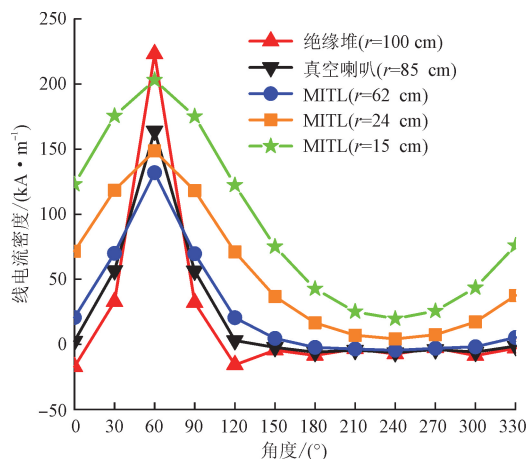
(b)不同位置的线电流密度
