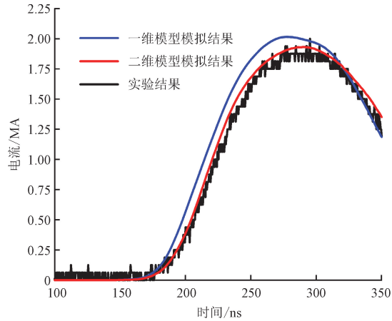
(b) 绝缘堆电流
