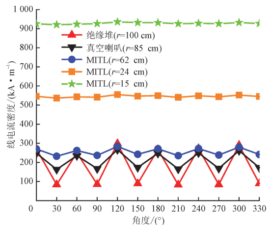
(b) 不同位置的线电流密度
