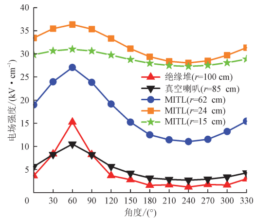
(a) 不同位置的电场
