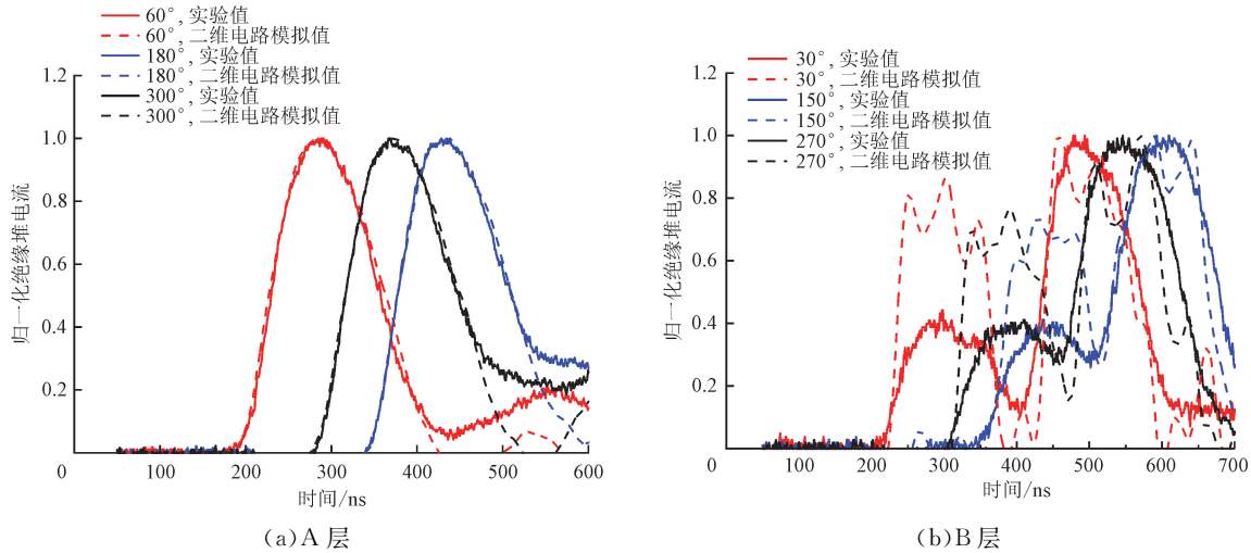
图9 不同角向位置的归一化绝缘堆电流波形
