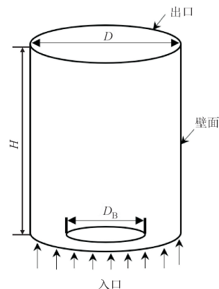
(a)垂直圆形截面管道几何模型
