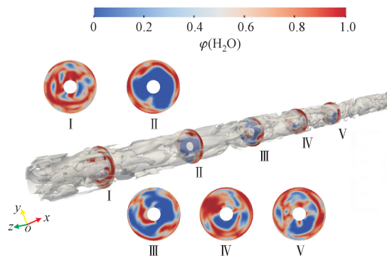
图 16 搅拌流等值面和径向截面两相分布
