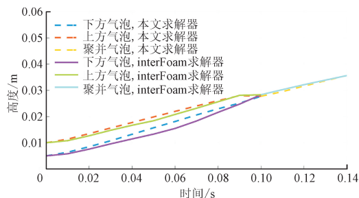
(b)双气泡质心高度随时间的变化
