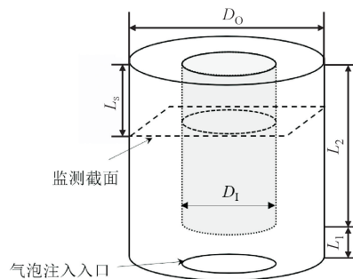
(a) 垂直环空几何模型
