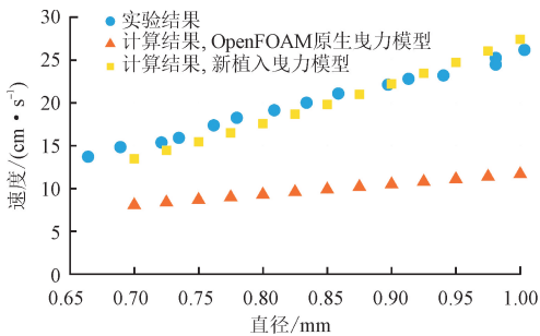
图 3 静水中单气泡上升终端速度计算结果与实验结果 [27] 的对比
