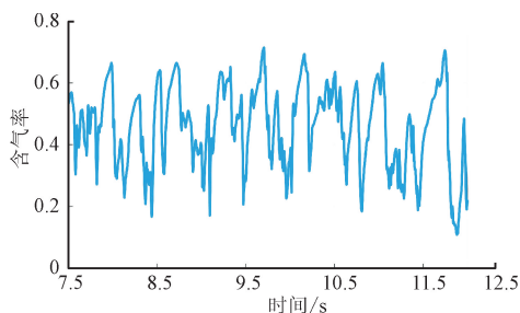
(a) 截面含气率
