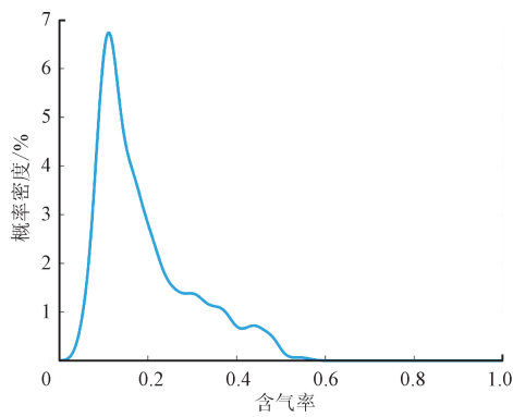
(b)截面含气率 PDF 分布
