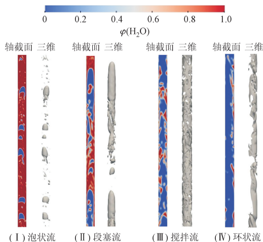
图 8 4 个选定工况下气液两相流型模拟结果
