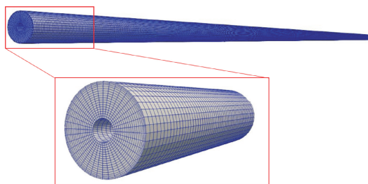
(b) 垂直环空网格模型
