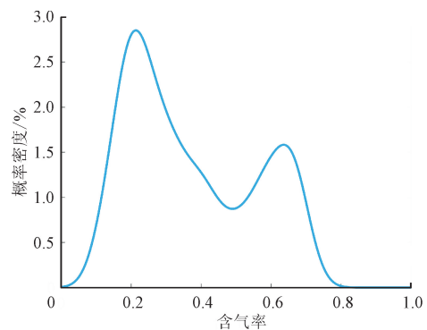
(b)截面含气率 PDF 分布
