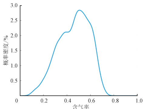
(b) 截面含气率 PDF 分布
