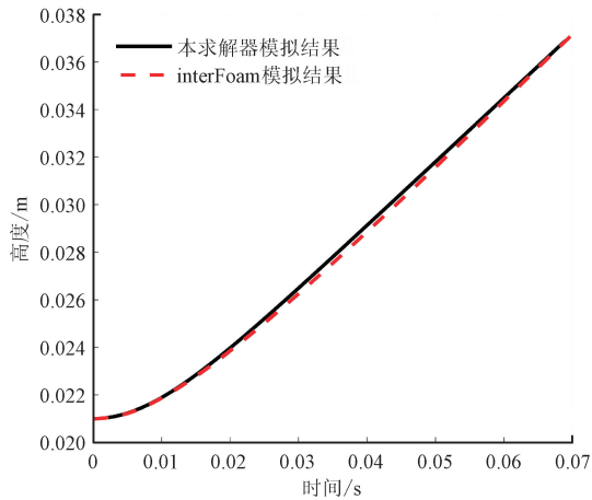
图 4 静水中单气泡上升过程数值模拟结果与 interFoam 模拟结果的对比
