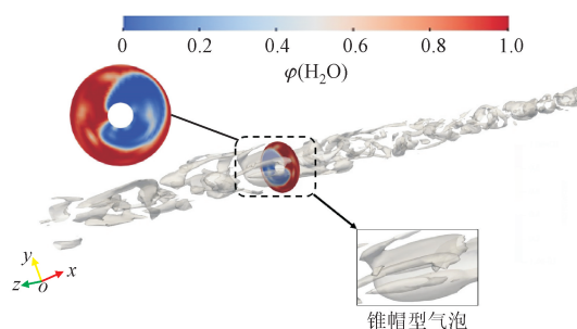
图 12 弹帽流等值面和径向截面两相分布
