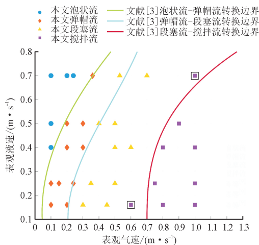
图 18 垂直环空气液两相流型图
