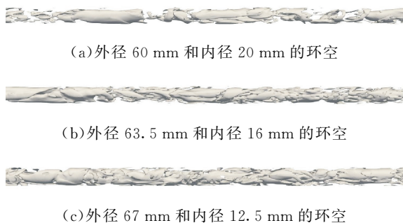
图 19 不同尺寸环空中气液两相等值面云图
