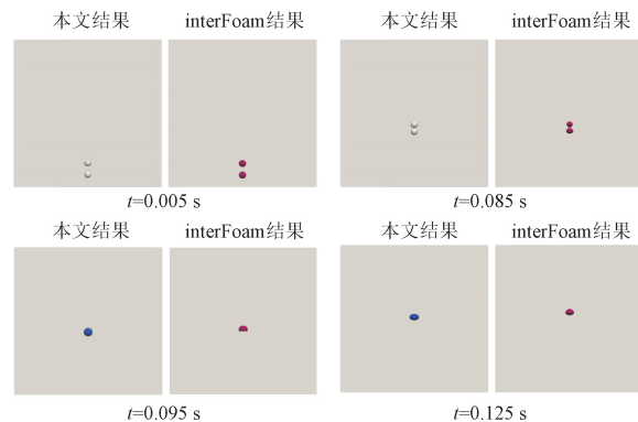
(a)典型时刻气泡形态和位置
