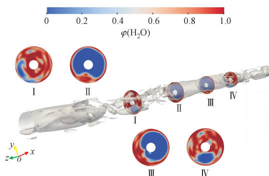
图 14 段塞流等值面和径向截面两相分布
