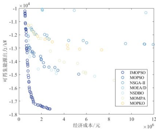
图6 IIES夏季典型日前沿
