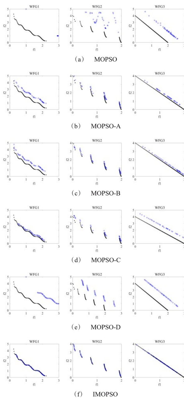
图3 消融实验结果
