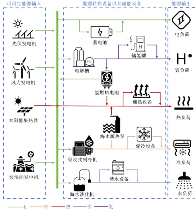
图1 IES系统结构示意图
