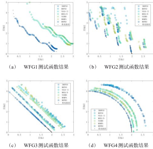
图4 WFG系列测试函数结果
