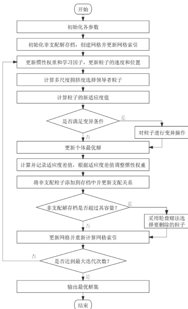
图2 IMOPSO 算法流程
