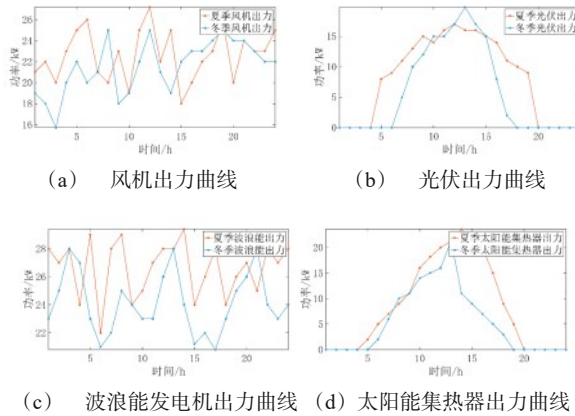
图5 可再生能源设备出力
