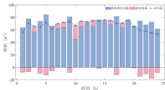
(d) IES水平衡
