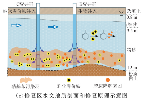
图7 原位化学-生物反应带修复硝基苯污染地下水工程概况示意图
