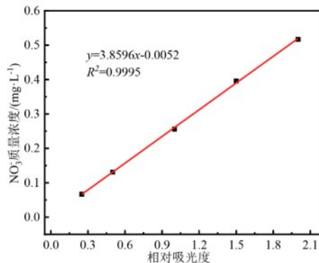
(c)溶液内 \text{NO}_3^- 标定曲线
