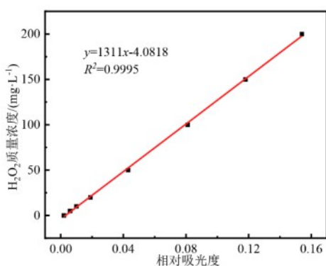
(a)溶液内 \text{H}_2\text{O}_2 标定曲线
