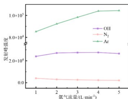
(b)随氩气流速提升时OH、N 2 和Ar的发射光谱
