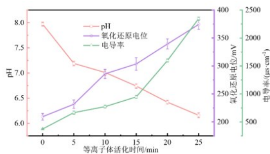
(a)等离子体活化水的pH值、ORP及电导率随等离子体活化时间的变化
