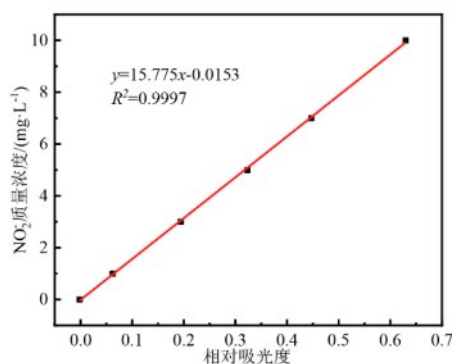
(b)溶液内 \text{NO}_2^- 标定曲线
