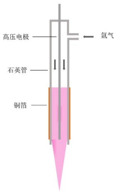
图1 实验装置示意图
