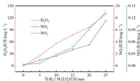
(b)等离子体活化水中 \text{H}_2\text{O}_2 、 \text{NO}_2^- 及 \text{NO}_3^- 浓度随等离子体活化时间的变化
