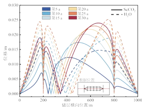
图6 不同工作介质分别在两井连接处引起的储层位移变化
