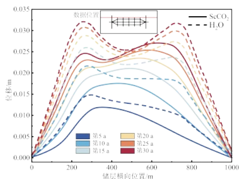
图5 不同工作介质分别在天然裂隙末端处引起的储层位移变化
