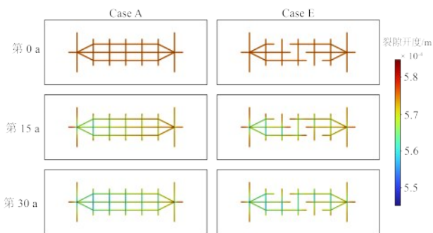
图 13 裂隙网络中的裂隙开度随时间变化
