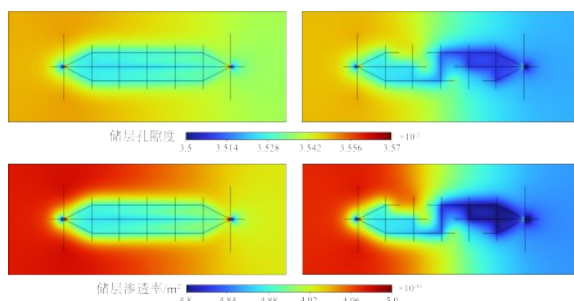
图 12 Case A 和 Case F 在第 30 a 时的储层孔隙度和渗透率
