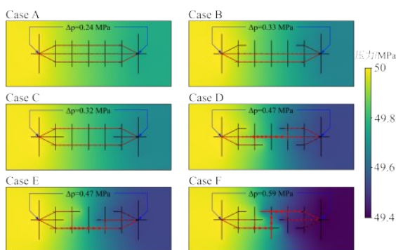
图 11 不同的多条水力裂隙网络在第 30 a 时的孔隙
