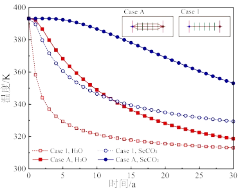
图3 不同工作介质下的生产井井底温度 Fig. 3 Bottomhole temperature of production wells under different working fluid
