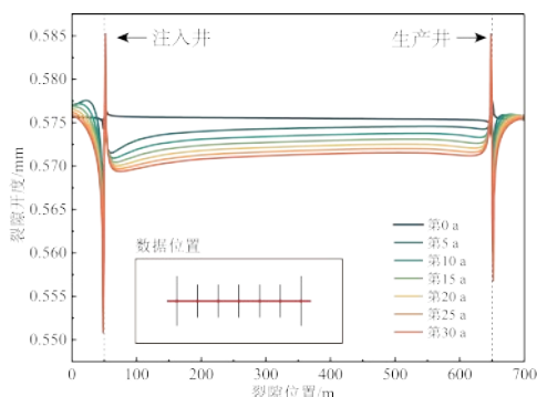
图 14 单水力裂隙网络下水力裂隙开度随时间的变化
