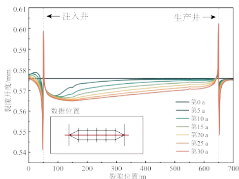
图 15 多水力裂隙网络下双井连接处水力裂隙
