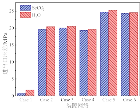
图4 不同工作介质和裂隙网络下第30 a 的储层流体
