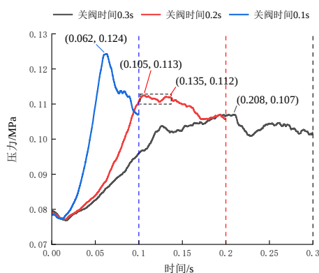
图16 不同关阀时间下水锤压力变化曲线
