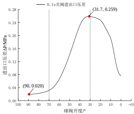
图9 球阀关闭过程进出口压差随开度变化曲线
