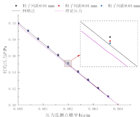
图6 MPS方法和网格法压力监测值与理论压力对比
