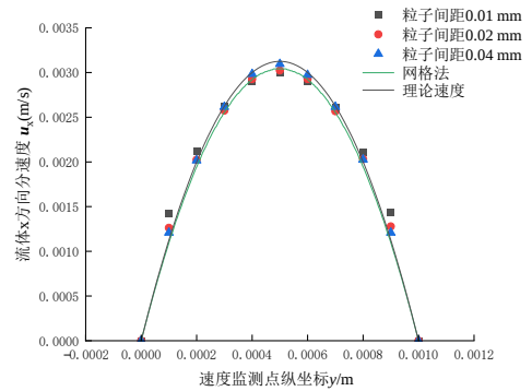
图4 MPS方法和网格法速度监测值与理论速度对比
