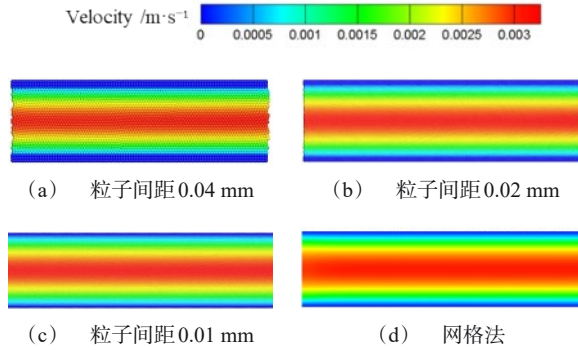
图3 泊肃叶流动速度云图
