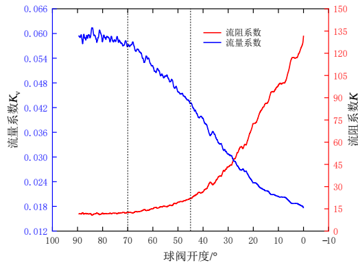
图 10 流量系数与流阻系数随开度变化曲线
