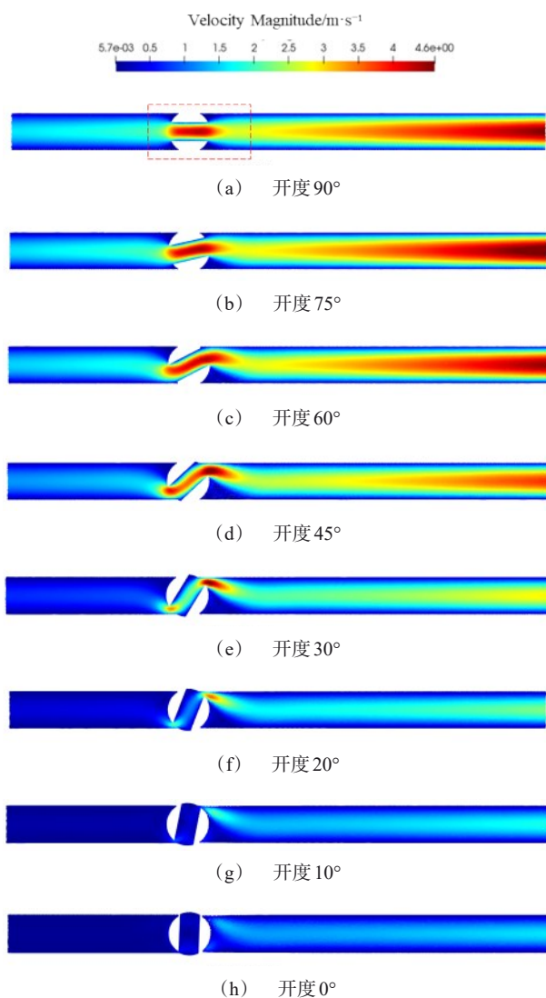
图 11 0.1 s 关阀过程不同开度下的球阀速度云图
