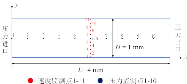
图2 算例几何布置
