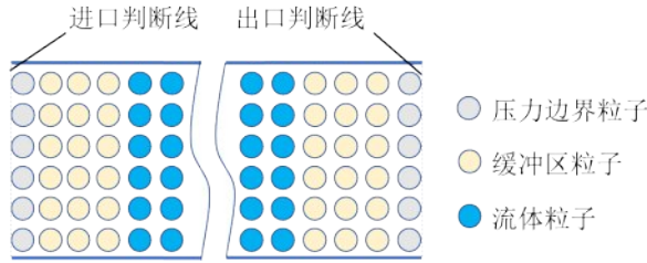
图1 压力进出口模型
