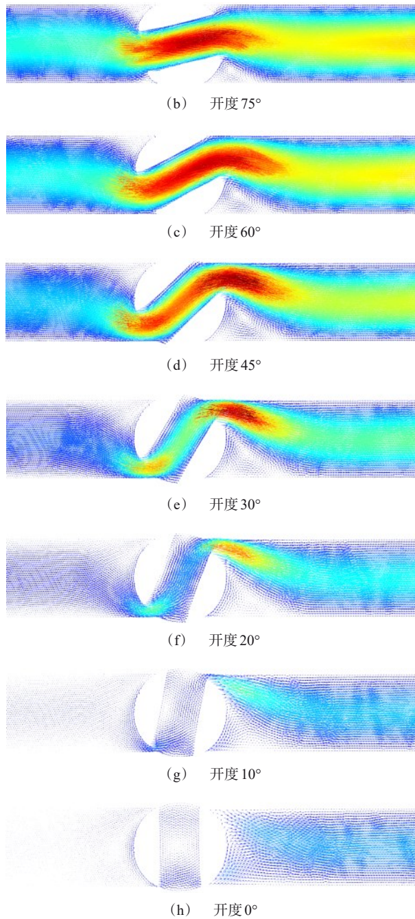
图12 0.1 s 关阀过程不同开度下的阀芯速度矢量图
