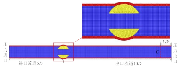
图8 球阀管道粒子离散图 Fig. 8 Ball valve pipeline particle discrete diagram
