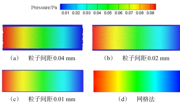
图5 泊肃叶流动压力云图
