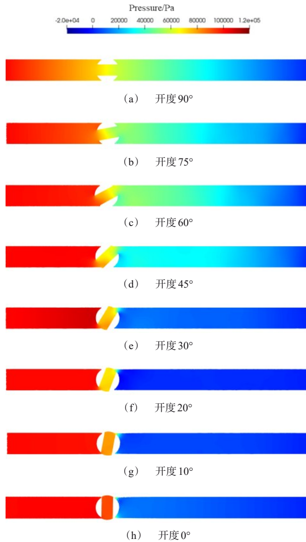
图 13 0.1 s 关阀过程不同开度下的球阀压力云图
