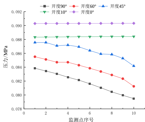
图15 0.1s 关阀过程不同开度下阀芯压力变化
